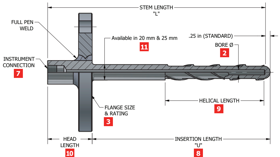
Helical Thermowell
